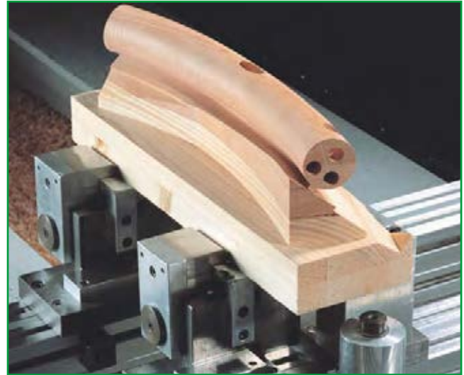
Bild 127/2: Horizontalspanner
