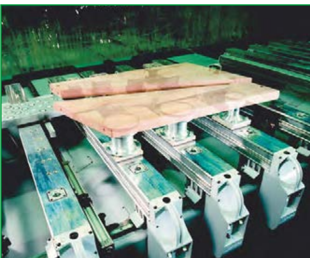
Bild 127/3: Stufentrennvorrichtung
