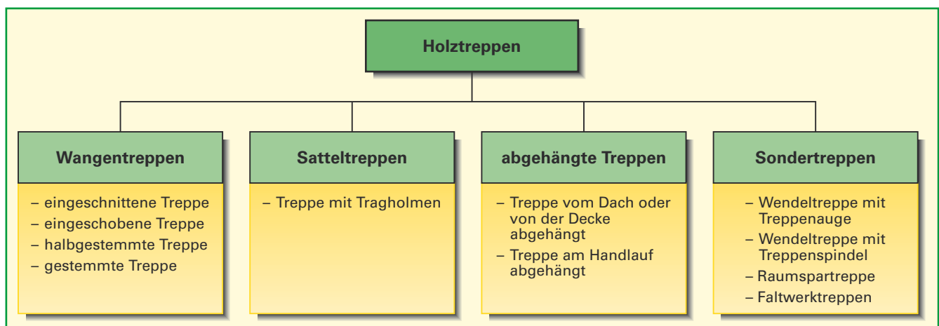
Bild 17/2: Bauarten von Holztreppe
