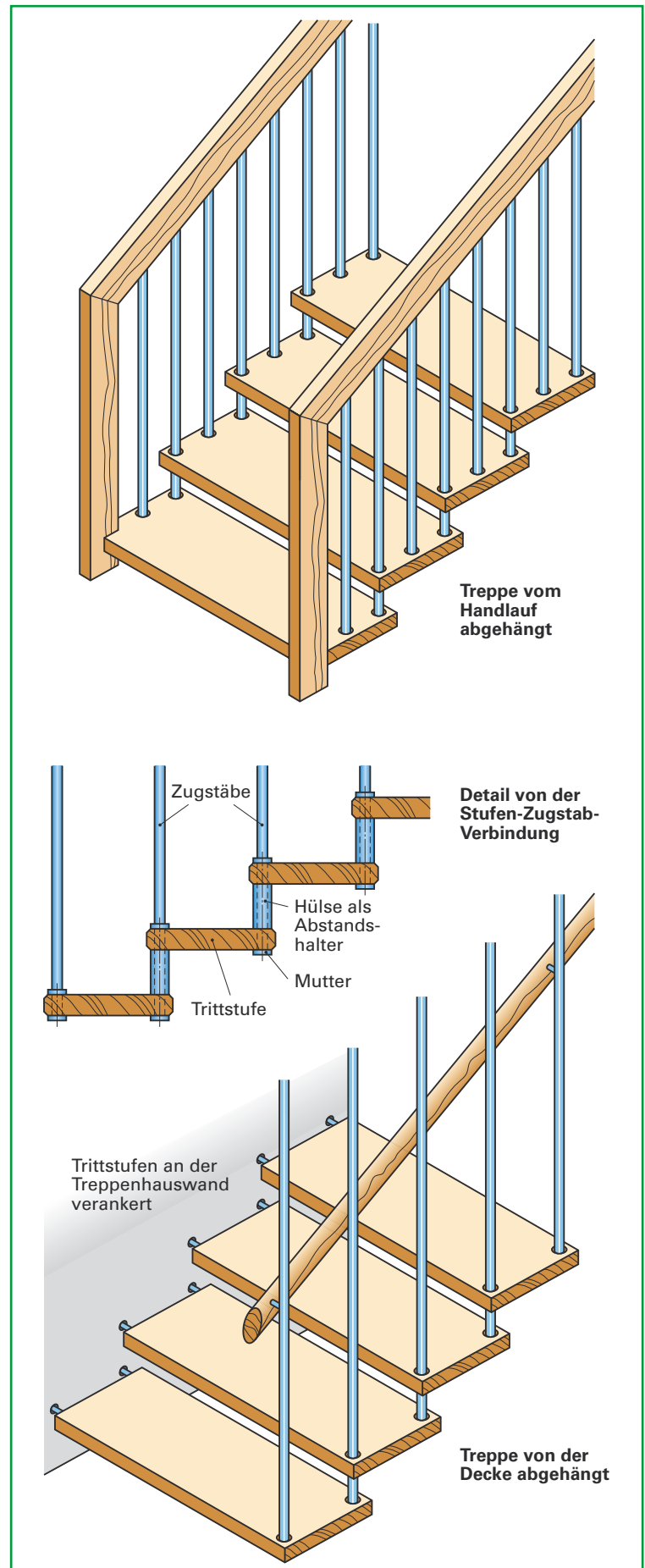
Bild 25/1: Abgehängte Treppen
