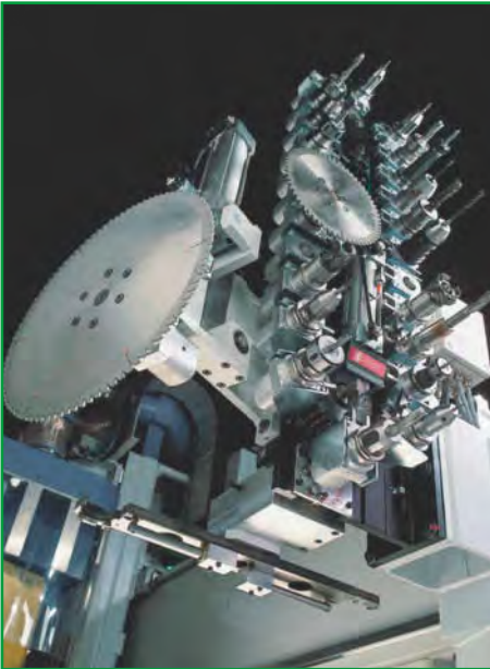
Bild 124/1: Kettenwechsler
